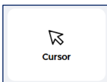
Figura 16. Botón Cursor
